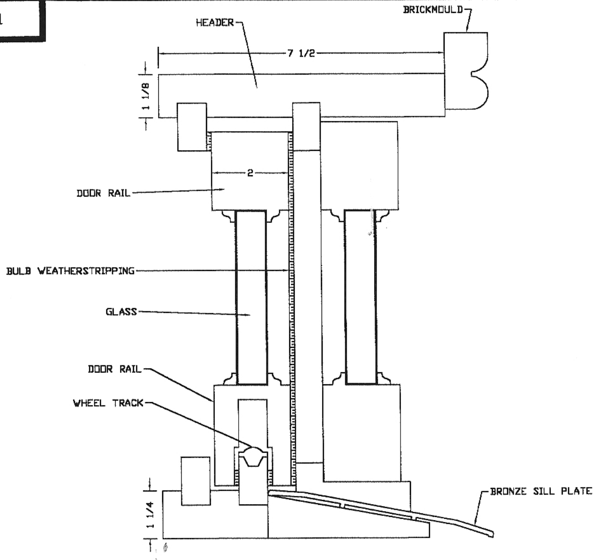
SLIDING DOOR HEADER & SILL DETAIL
